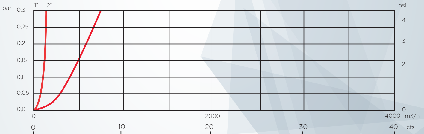
DESCARGA DE AIRE DURANTE EL LLENADO DE LA TUBERIA
